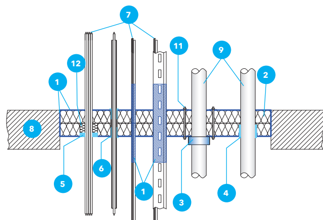
Detalle B Multipenetración en forjado
