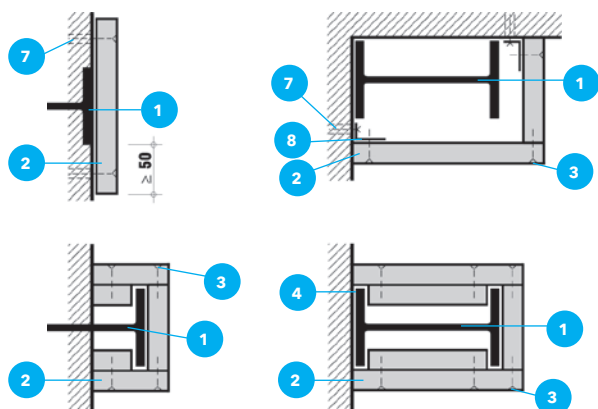
Detalles para fijación a una, dos y tres caras
