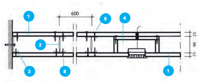
DETALLE 2: CORTE EN SECCIÓN CON SELLADO DE TUBERÍAS Y REGISTRO
