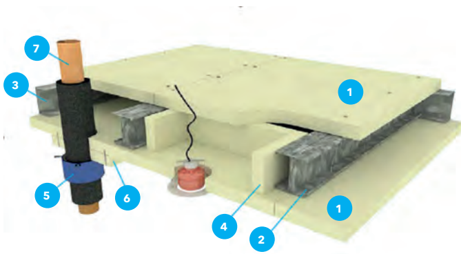
DETALLE 1: CORTE EN SECCIÓN Y LUMINARIA
