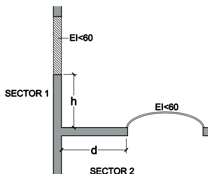
Figura 2.1 Encuentro cubierta - fachada.
