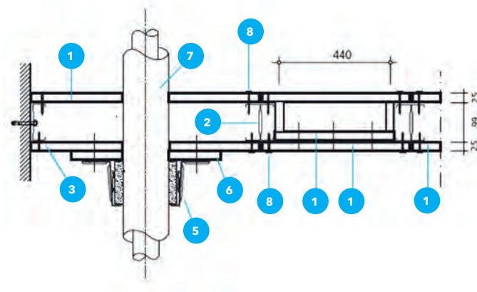
DETALLE 2: CORTE EN SECCIÓN CON SELLADO DE TUBERÍAS Y REGISTRO
